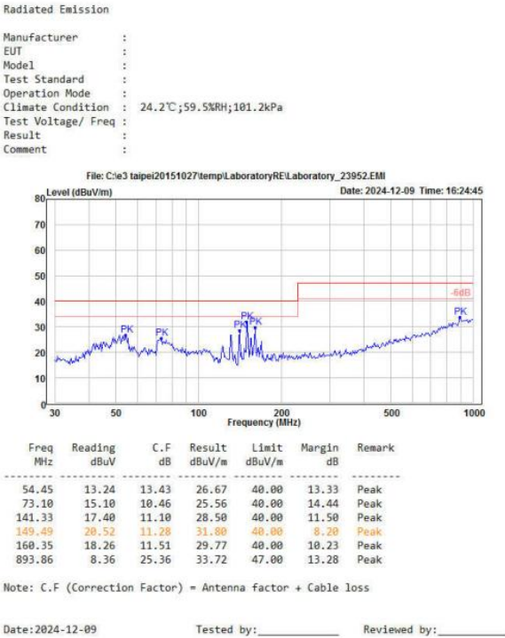
图 6-7 辐射测试垂直方向
