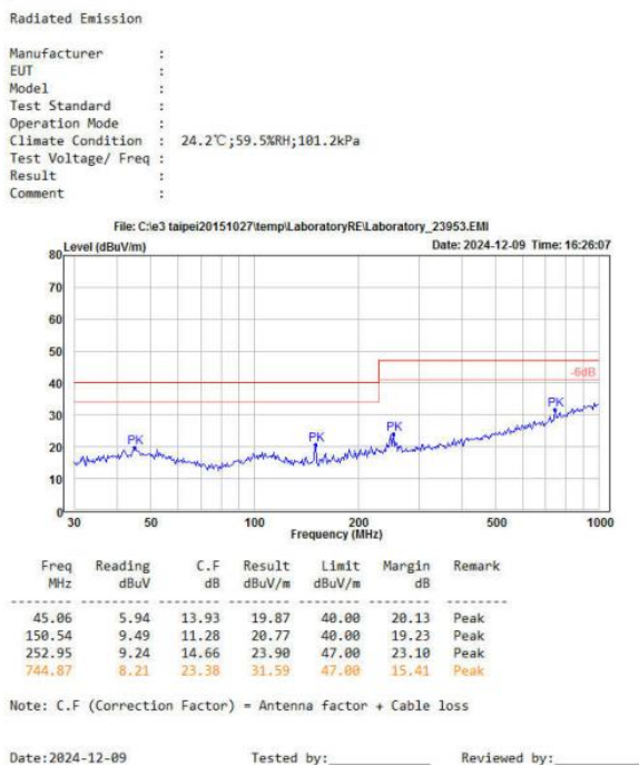
图 6-6 辐射测试水平方向
